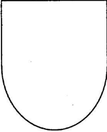
Darah'ın Şekli
